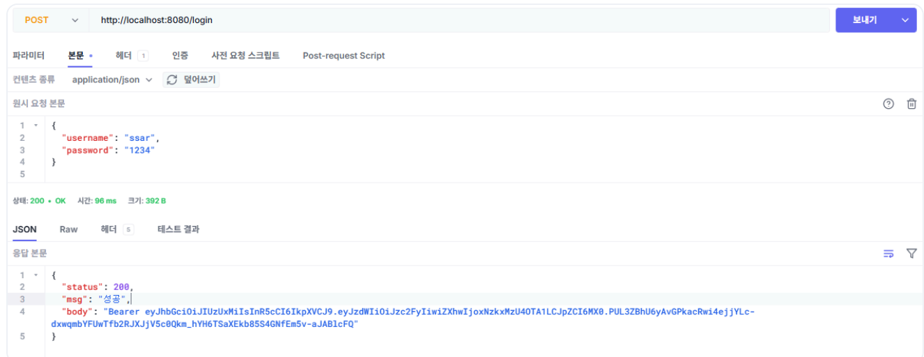
그림 4-14. 로그인 응답
